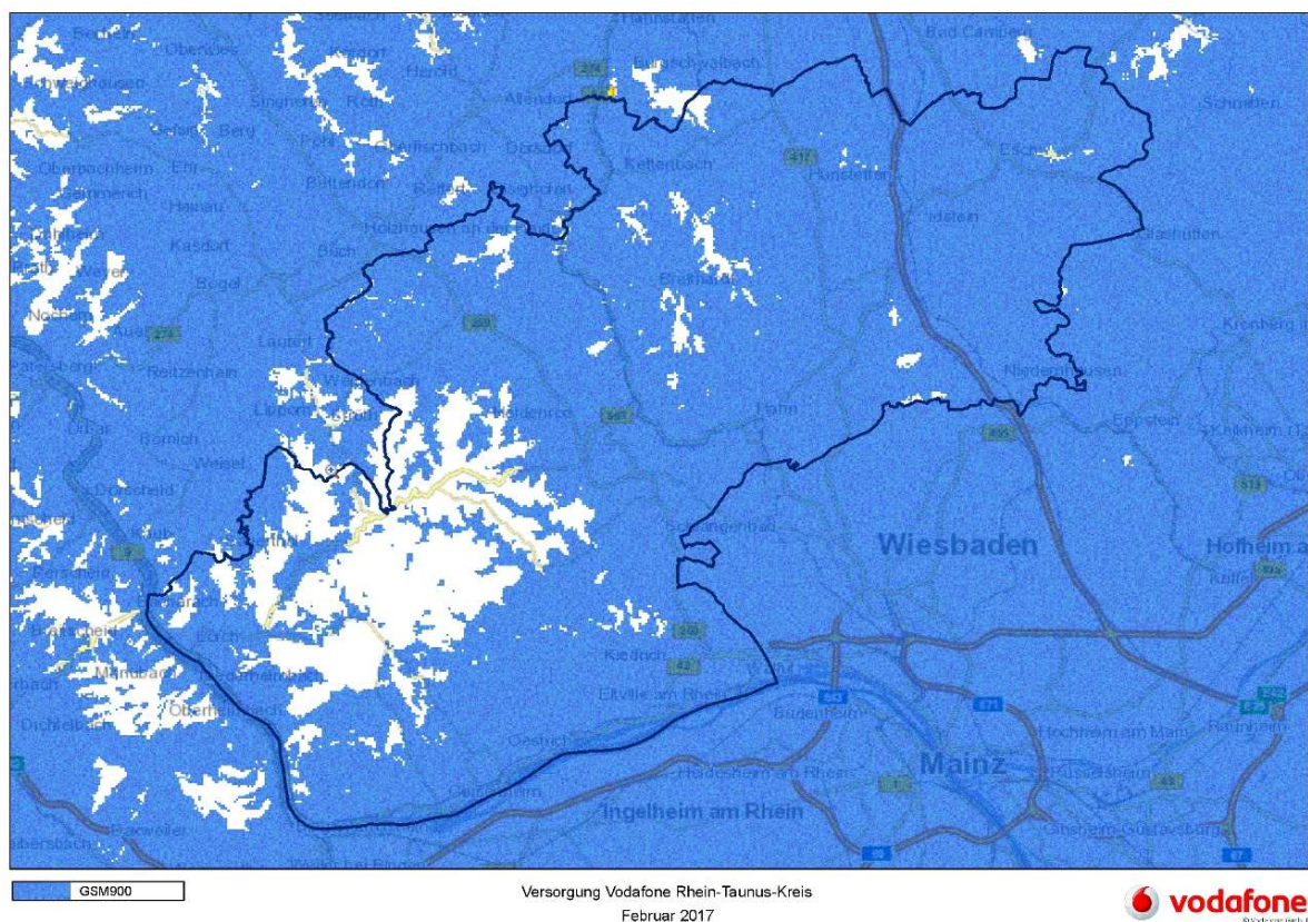
Grafik 7: GSM-Versorgung von Vodafone im Rheingau-Taunus-Kreis, Quelle: Vodafone GmbH, Stand: Februar 2017
