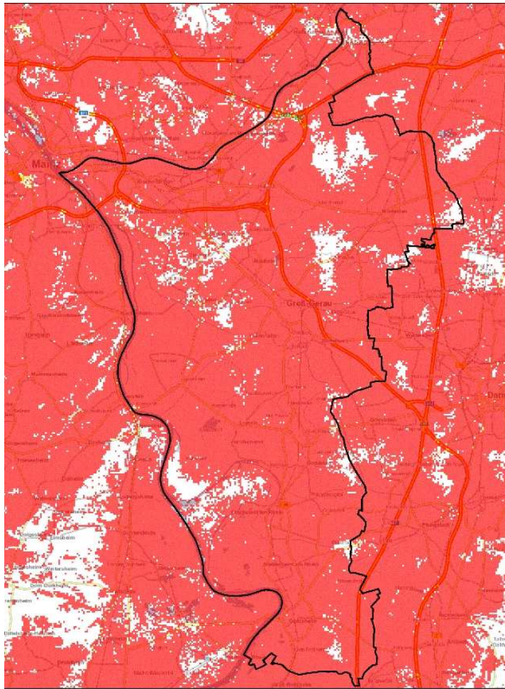
Grafik 9: LTE-Versorgung von Vodafone im Landkreis Groß-Gerau, Quelle: Vodafone GmbH, Stand: August 2017
