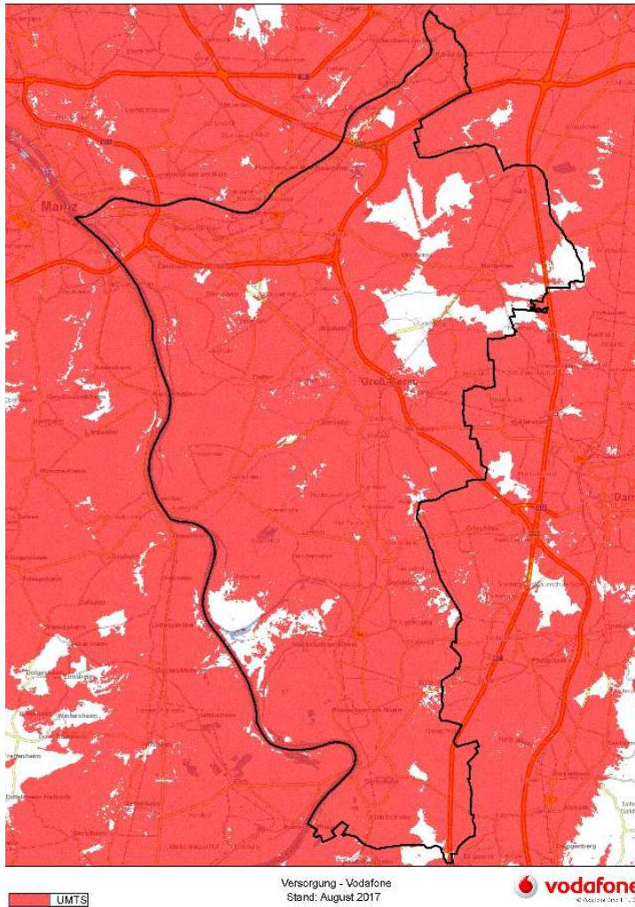
Grafik 8: UMTS-Versorgung von Vodafone im Landkreis Groß-Gerau, Quelle: Vodafone GmbH, Stand: August 2017
