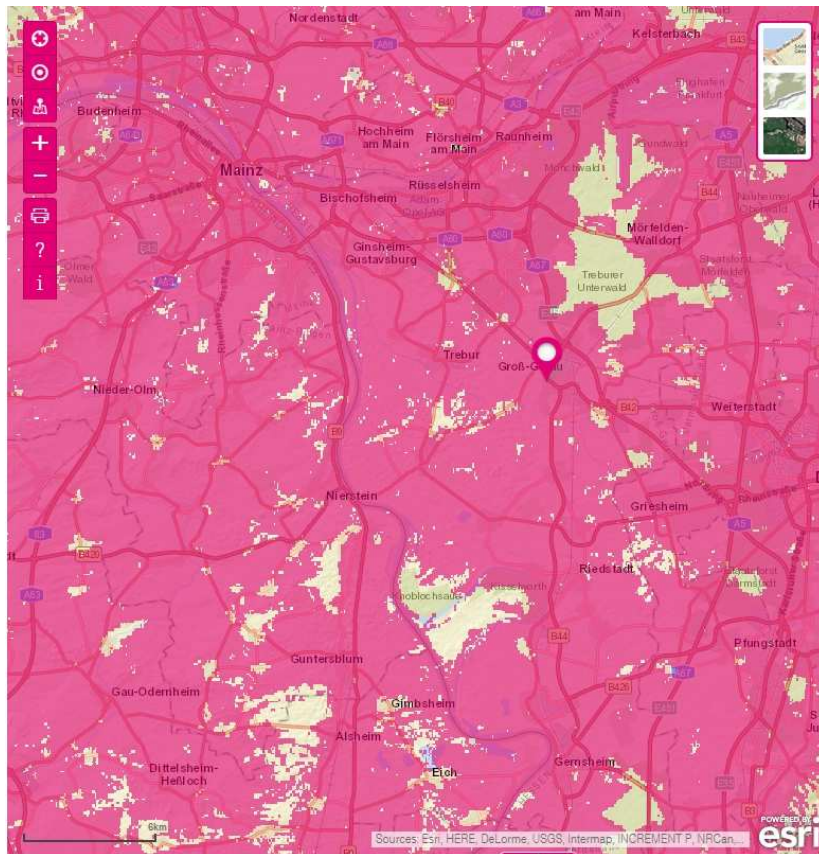
Grafik 2: UMTS-Versorgung der Deutschen Telekom im Landkreis Groß-Gerau, Quelle: www.telekom.de/netzausbau , Stand: September 2017
