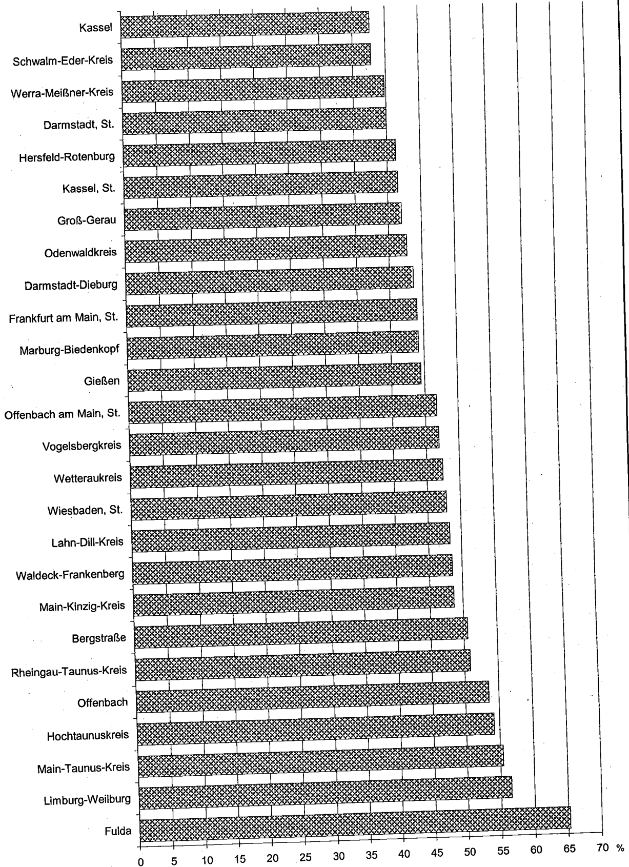
Rangfolge der Stimmenanteile der CDU
